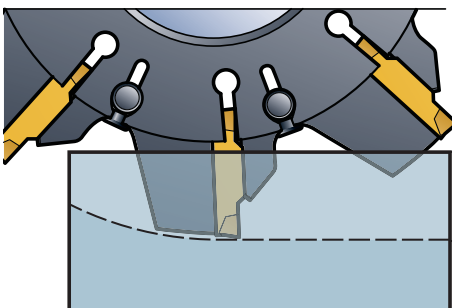
Maximale Schnitttiefe (mm)
